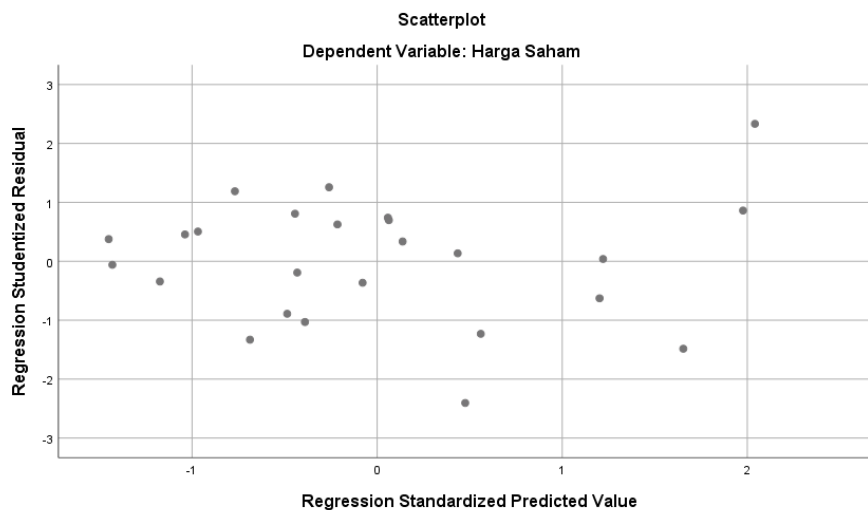
Gambar 4.1 Grafik Scatterplot
